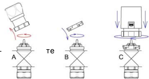
Рис 2. Монтаж сервоприводов
