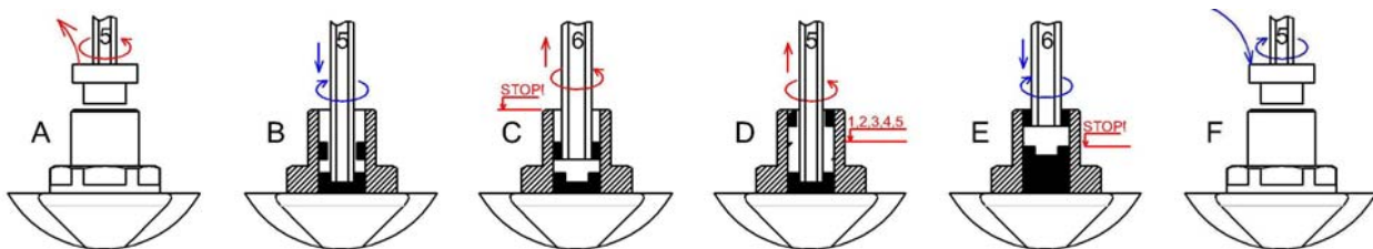
Рис 5 балансировка коллектора
