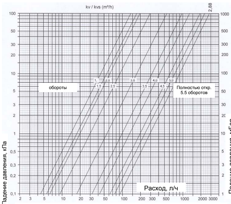
Рис.6. Номограмма падение давления/расход для балансировочных клапанов.
